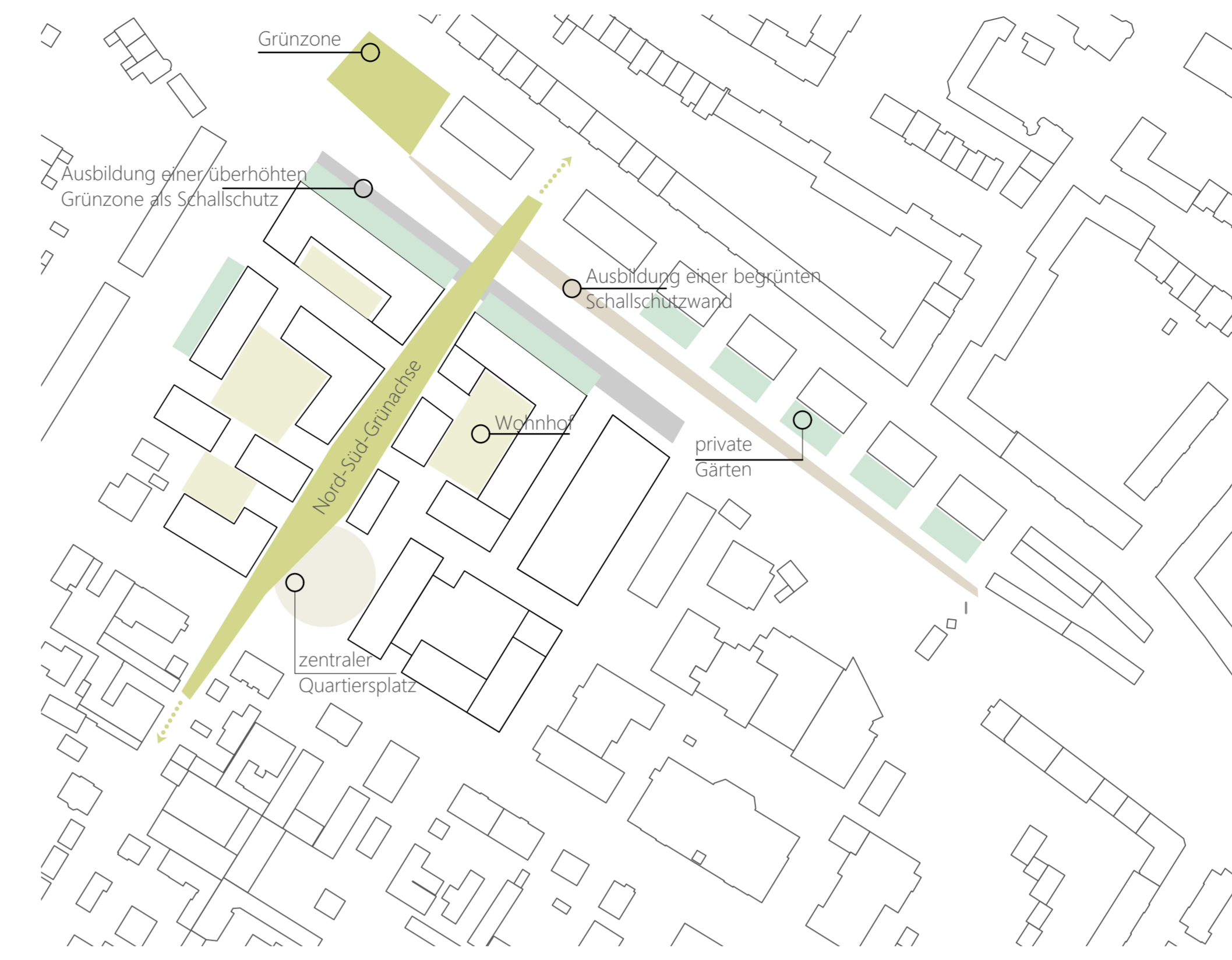
Freiraum / Grünkonzept
