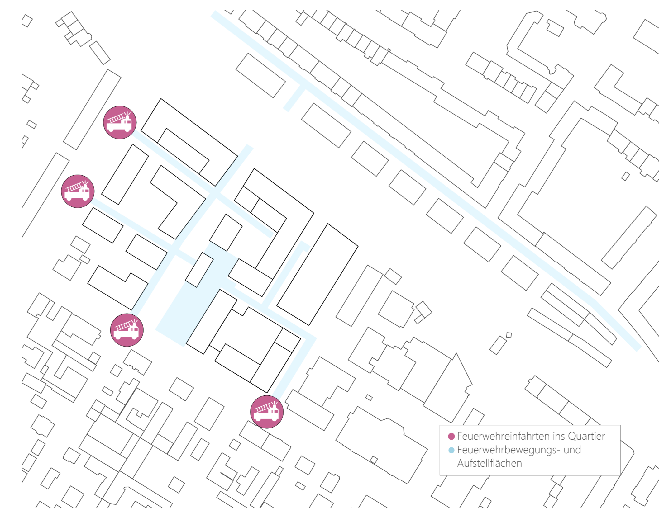
Feuerwehraufstellflächen
