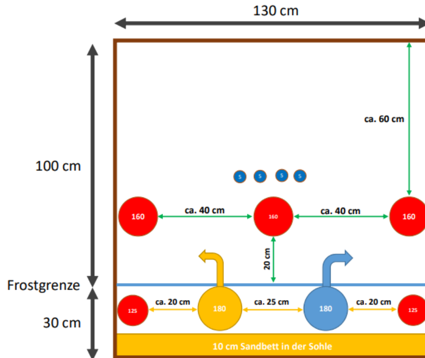
Rohrgrabenprofil: Zwischen beiden Sielen
